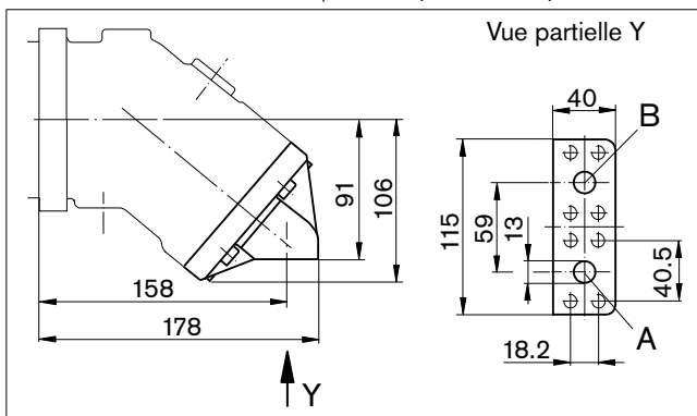
10 – Raccords à bride SAE, en bas (même côté) 4)
