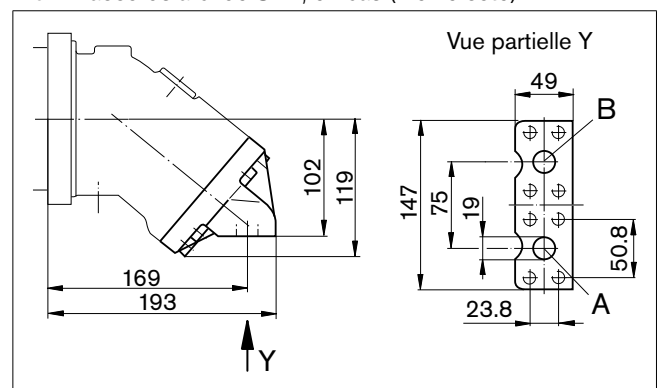
10 – Raccords à bride SAE, en bas (même côté)
