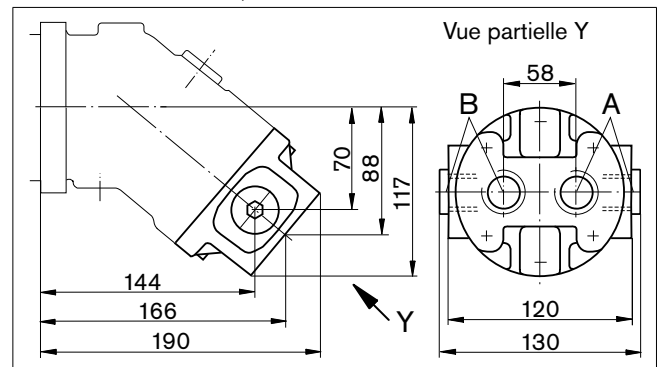
04 – Raccords filetés, latéral et arrière
