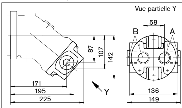
04 – Raccords filetés, latéral et arrière
