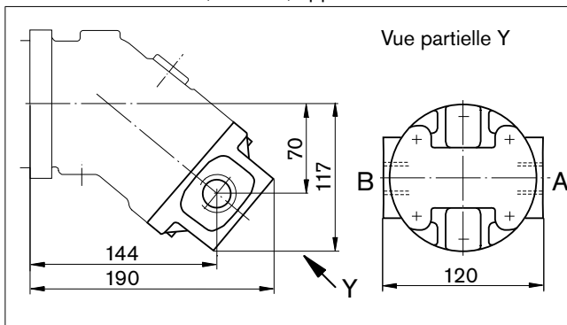
03 – Raccords filetés, latéraux, opposés
