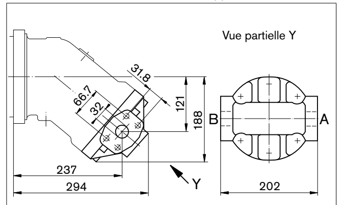
02 – Raccords à bride SAE, latéraux, opposés
