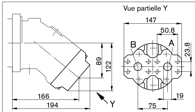
01 – Raccords à bride SAE, à l'arrière
