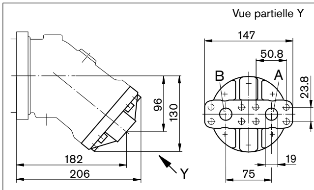
01 – Raccords à bride SAE, à l'arrière
