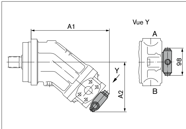
Plaque de raccordement 027 – Raccords à bride SAE, latéraux
