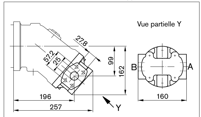
02 – Raccords à bride SAE, latéraux, opposés
