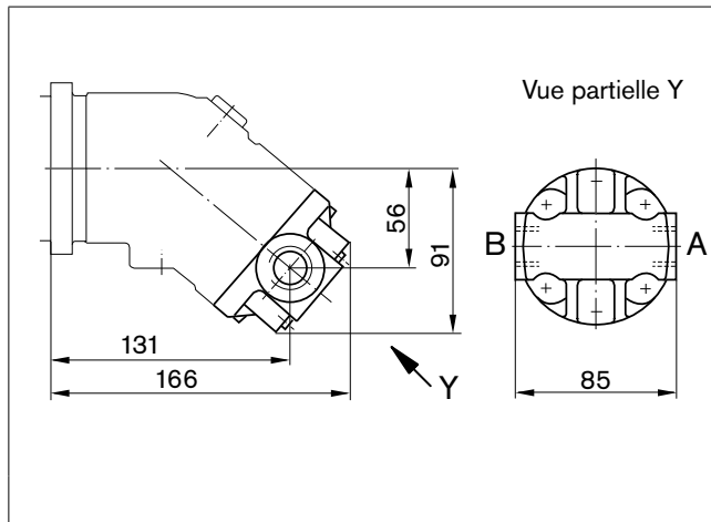
03 – Raccords filetés, latéraux, opposés
