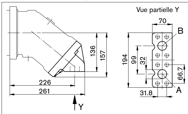
10 – Raccords à bride SAE, en bas (même côté)
