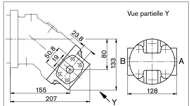
02 – Raccords à bride SAE, latéraux, opposés
