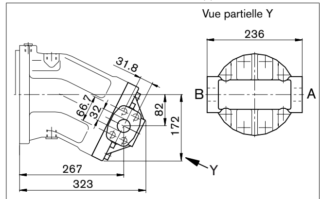
02 – Raccords à bride SAE, latéraux, opposés
