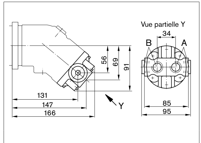
04 – Raccords filetés, latéral et arrière
