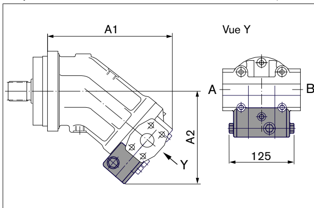
Plaque de raccordement 029 – Raccords à bride SAE, latéraux
