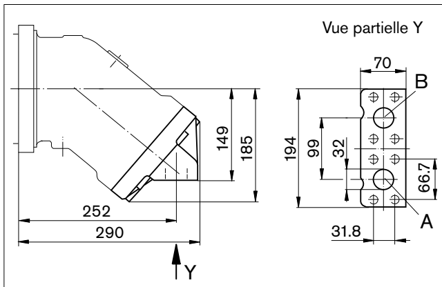
10 – Raccords à bride SAE, en bas (même côté)
