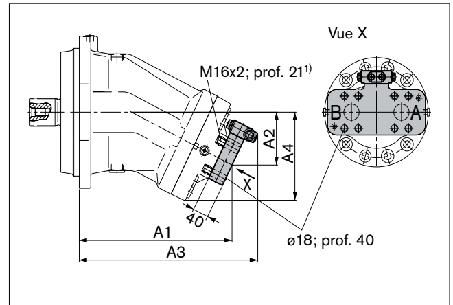
Plaque de raccordement 017 – Raccords à bride SAE, à l'arrière
