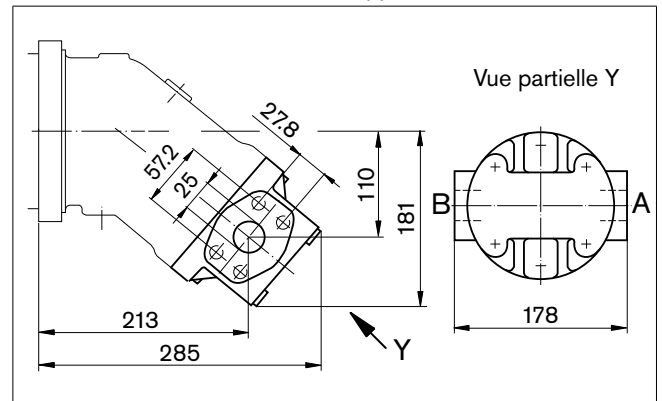
02 – Raccords à bride, latéraux, opposés (taille 107)
