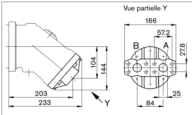
01 – Raccords à bride SAE, à l'arrière
