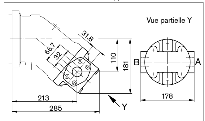
02 – Raccords à bride, latéraux, opposés (taille 125)
