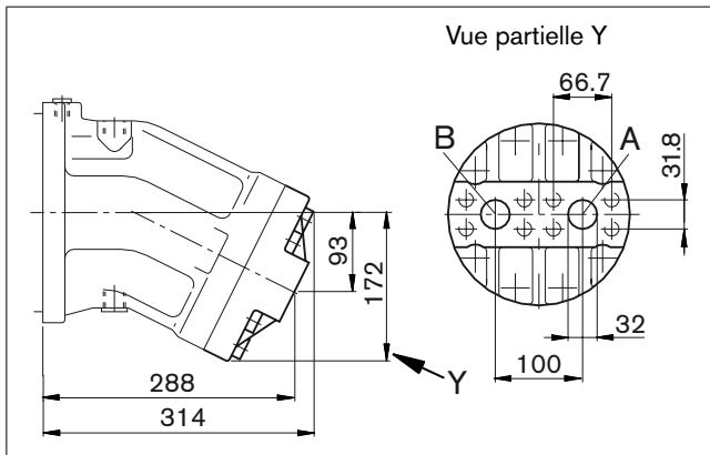
01 – Raccords à bride SAE, à l'arrière
